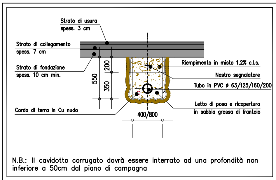
PARTICOLARE SEZIONE SCAVO E POSA CAVIDOTTI BT (tipico)
